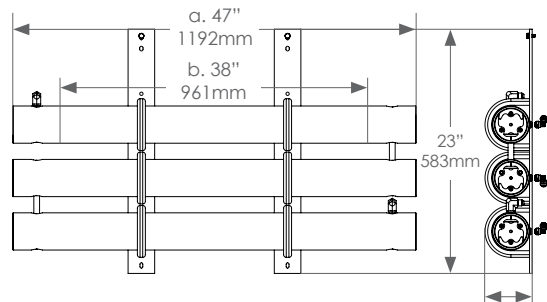
Vessel Assembly a: 2700 / 3200 / 3400 b: 2100 / 2600
